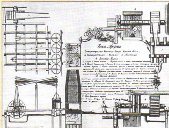
Чертеж оборудования Екатеринбургского завода. Первая половина XIX в.
